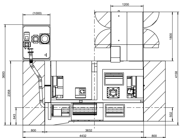
Layout CamGrind L1, 650 mm Spitzenweite
